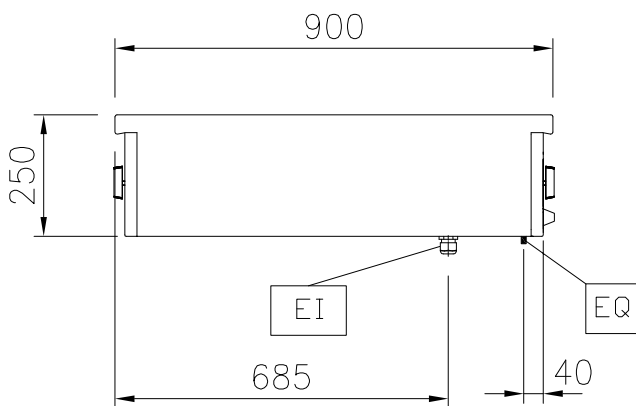
Zij aanzicht
