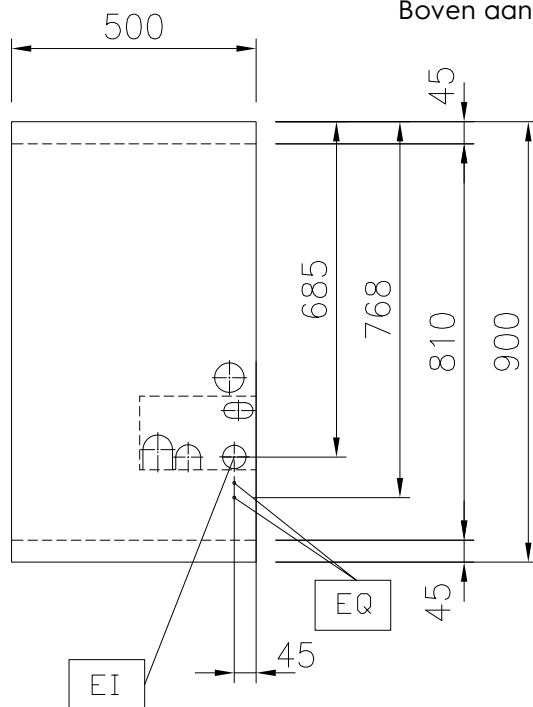
Boven aanzicht
